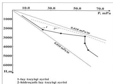
Şəkil 2. Kürəvdağ yatağında lay təzyiqlərin dərinlikdən asılı olaraq dəyişməsi
