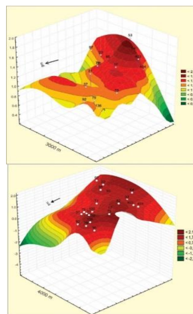
Şəkil 1. Kürsəngə yatağının 3000 və 4000 m dərinlik kəsilişində anomaliya
